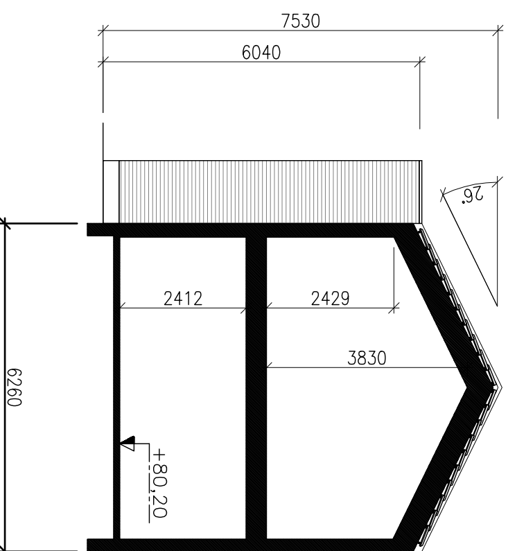
SNITT AA
